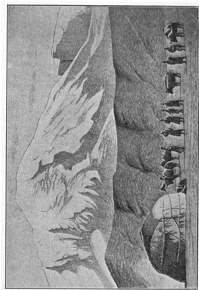
Высочайшая вершина Мустагъ-агы; видъ съ запада. (Съ плоскогорья агора).
