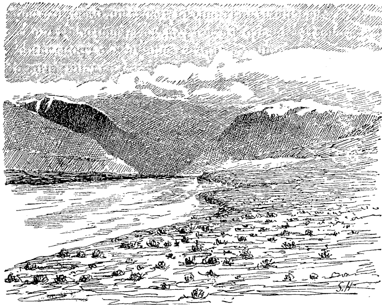
р. Ики-бель-су. Видъ на юго-востокъ.
