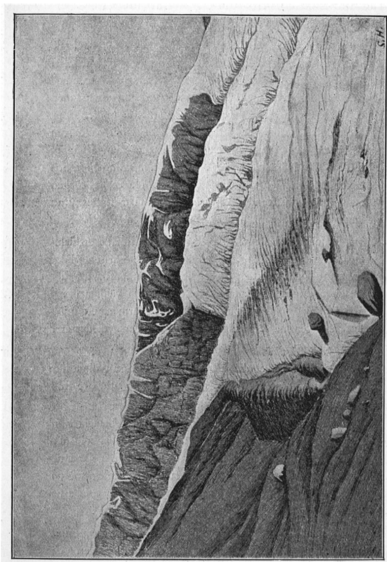
Мѣсто слиянія трехъ рукавовъ ледника Тергенъ-булака. (Съ рисунка автора).
