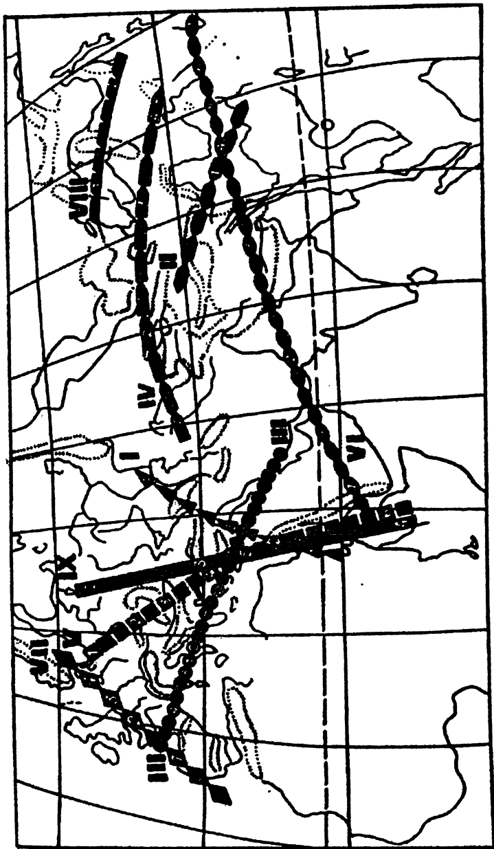
Рис. 2. Оси зон пассионарных толчков
