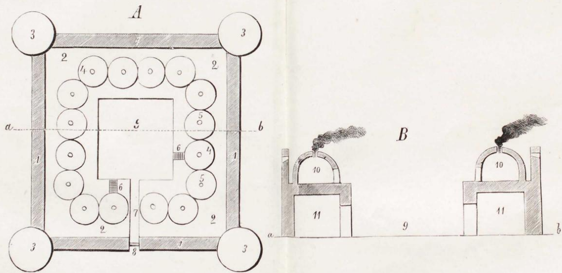
A. Планъ селенія Шормасть; B. Профиль по линіи ab ; 1) наружная стѣна; 2) крыша нижняго этажа, на которой поставлены куполообразные жилые дома; 3) башня; 4) куполообразные жилые дома; 5) отверстіа для дыма; 6) лѣстница; 7) проходъ; 8) ворота; 9) общій видъ; 10) жилой домъ; 11) нижній этажъ для скота.
