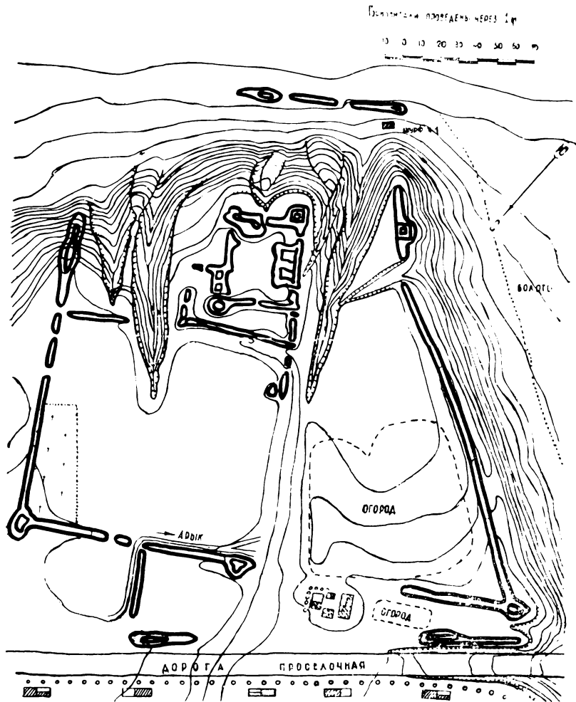
План киргизско-кокандского укрепления Улу-Коргон XVIII—XIX вв. Сост. Е. З. Заурова, 1969 г.
